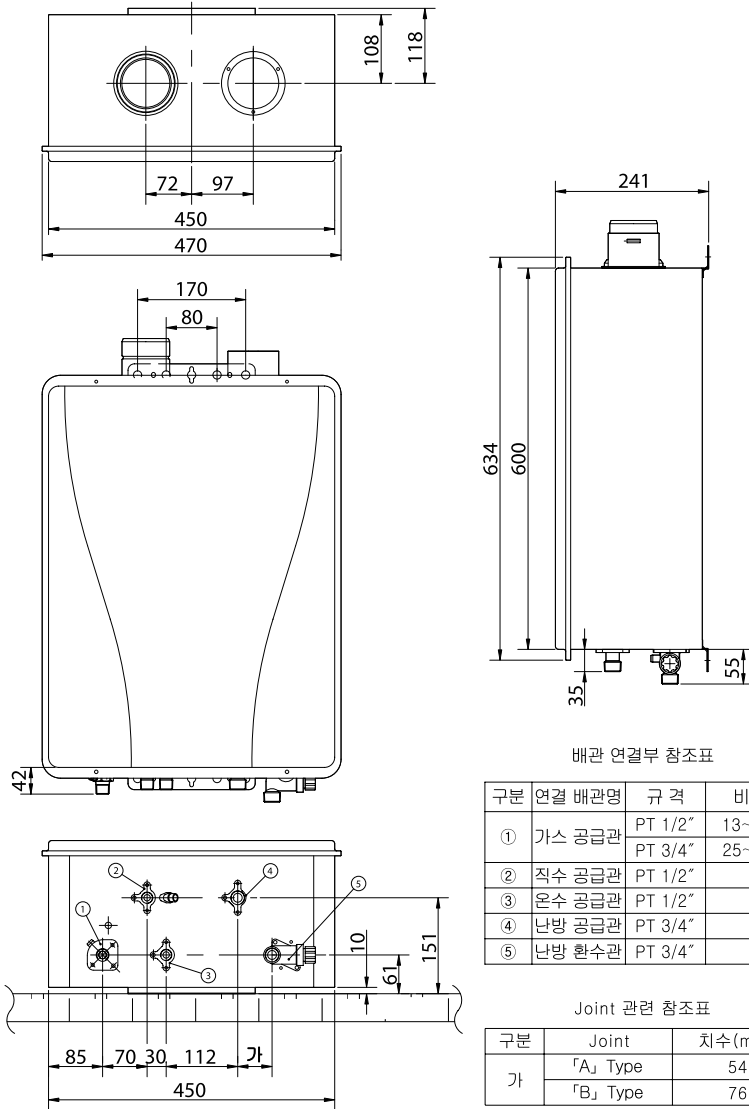
외관도(13~35K)
